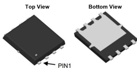
PDFN5X6-8L
